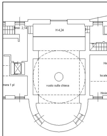
Fig. 7 - Pianta piano primo
