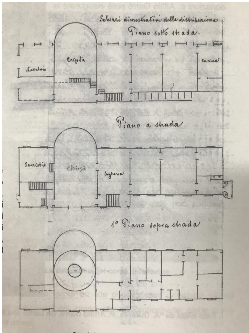
Fig. 3 - Pianta dell'edificio allegata a una perizia del 1924
