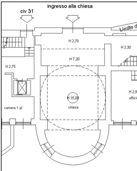
Fig. 6 - Pianta piano terra
