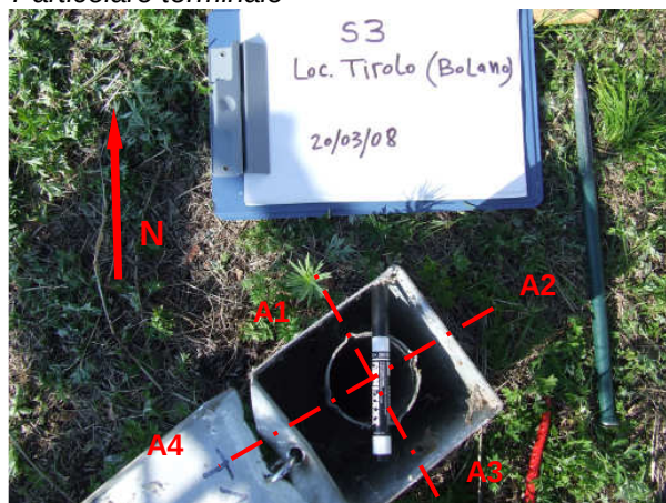
Particolare terminale
