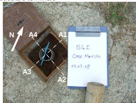
Particolare terminale
