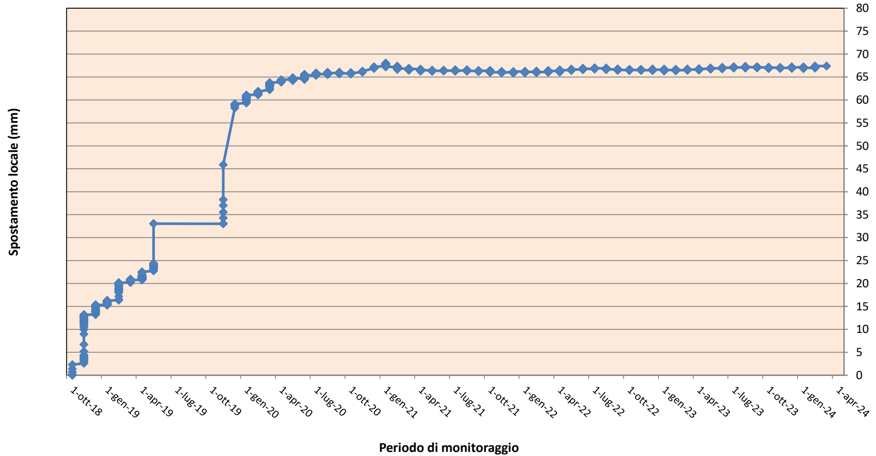
Sito Sant'Olcese - sonda automatica in SOLS4 - (profondità -12,5m)
